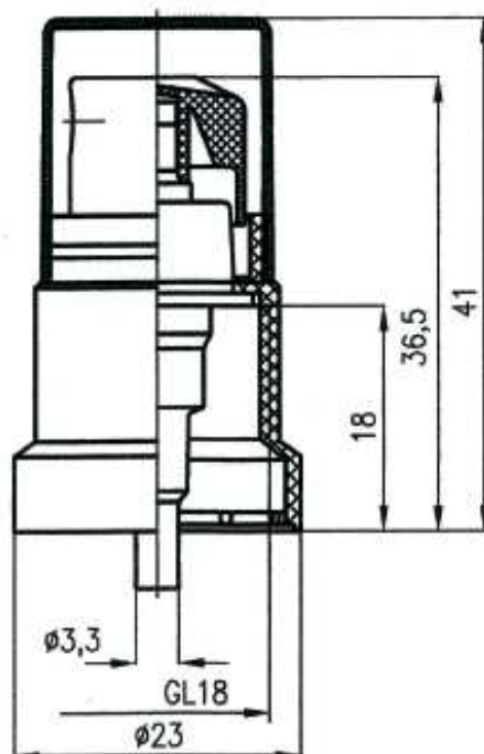
Jednočinný mechanický rozprašovač pro malé dávky média
